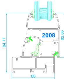
Marco estándar Hoja de ventana estándar
