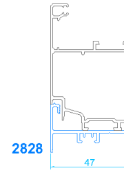
Perfil hoja marco abierto
