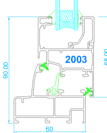
Marco estándar Hoja de ventana ajunquillada
