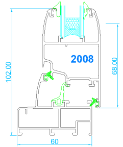
Marco ventana Hoja apertura exterior sin junquillo
