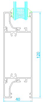
Zócalo marco abierto
