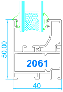
Marco para fijo de 40
