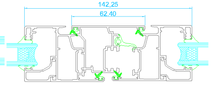
Nudo central Unión hojas ajunquilladas
