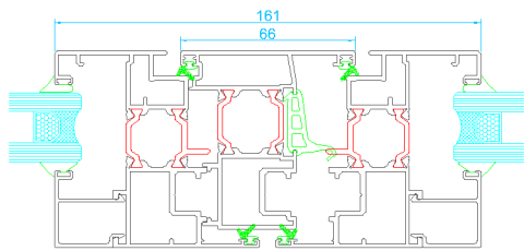
Unión hojas e inversora
