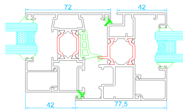
Unión hoja y travesaño
