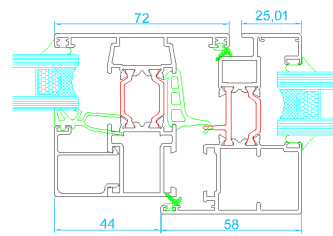
Unión hoja y travesaño
