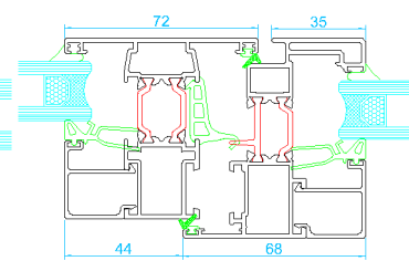
Unión hoja ajunquillada y travesaño
