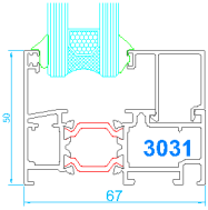
Marco para fijo
