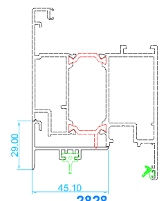
Perfil hoja marco abierto
