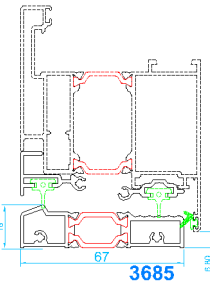
Marco reducido Hoja balconera
