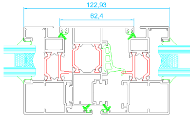
Unión hojas nudo central
