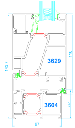
Marco balconera Hoja balconera apertura exterior
