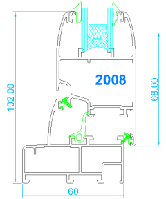
Marco ventana Hoja apertura exterior sin junquillo
