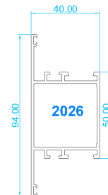
Travesaños
