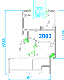
Marco estándar Hoja de ventana ajunquillada
