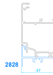
Perfil hoja marco abierto
