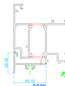
Perfil hoja marco abierto
