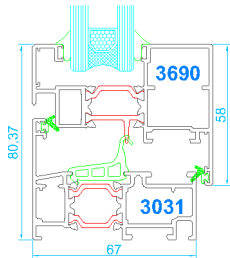
Marco estándar Hoja de ventana
