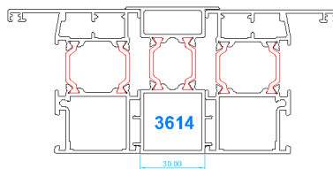
Perfil de unión inercia
