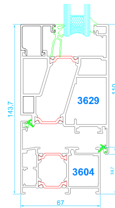
Marco balconera Hoja balconera apertura exterior
