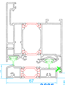
Marco reducido Hoja balconera
