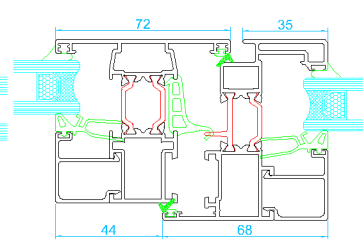
Unión hoja ajunquillada y travesaño
