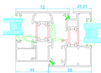
Unión hoja y travesaño
