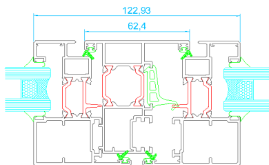
Unión hojas nudo central
