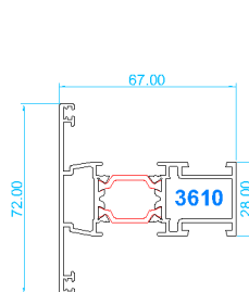
Perfil de unión inercia
