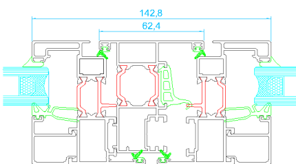
Unión hojas ajunquilladas nudo central
