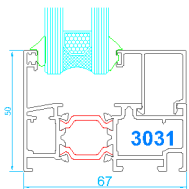
Marco para fijo
