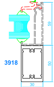
Cruce con refuerzo de inercia
