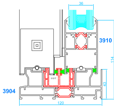
Marco de corredera Hoja de corredera
