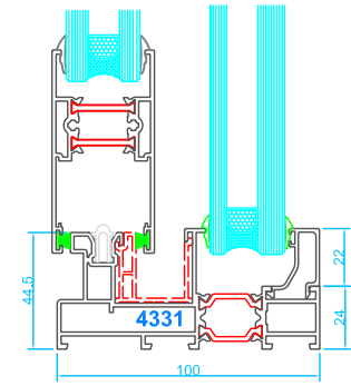
Marco de corredera con 1 hoja fija
