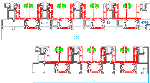
Marco multicarril, posibilidad infinita de hojas
