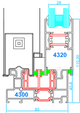
Marco de corredera Hoja de corredera
