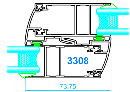
Bajo petición Cruce perimetral Combinado con hoja perimetral
