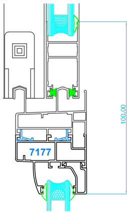
Unión invisible marco corredera con fijo
