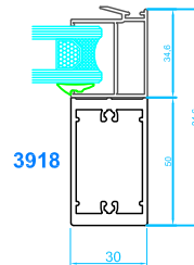
Cruce con refuerzo de inercia
