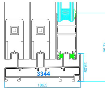
Marco de corredera de triple caril Hoja de corredera
