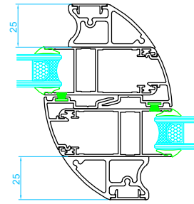
Cruce con refuerzo de inercia
