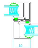
Cruce minimalista Combinado con hoja corte recto
