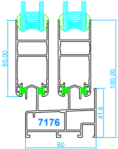
Marco de corredera Hoja perimetral
