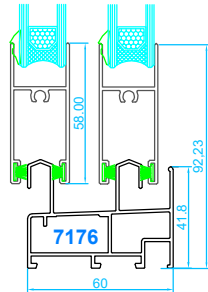
Marco de corredera Hoja corte recto
