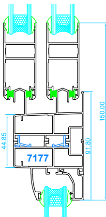
Unión invisible marco corredera con fijo
