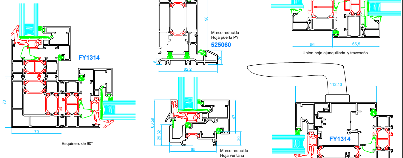
Acople en hoja oculta para cerradura marco ventana
