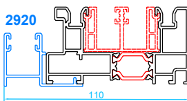
Guía de persiana especial reducida
