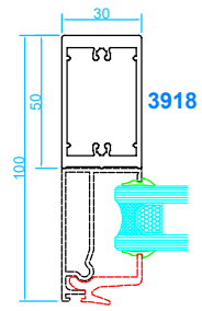
Cruce con refuerzo de inercia
