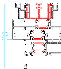
Unión marco corredera con fijo
