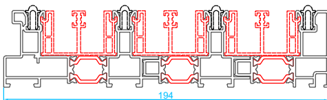
Marco 4 carriles, posibilidad de marcos combinables, hasta 12 carriles.
