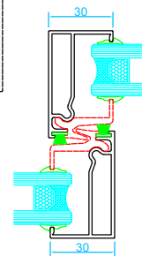
Cruce estándar
