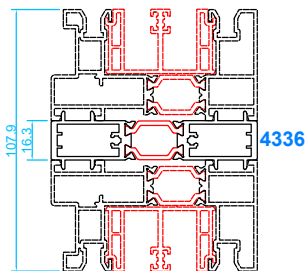
Unión marco con marco corredera
