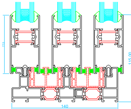
Marco de corredera de triple carril Hoja de corredera
