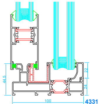
Marco de corredera con 1 hoja fija
