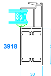
Cruce con refuerzo de inercia
