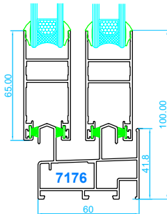
Marco de corredera Hoja de corredera
