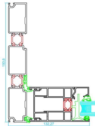
Marco de corredera 3 carriles sección lateral Hoja de corredera
