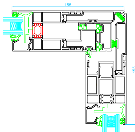
Encuentro en esquina 90° sin parteluces
