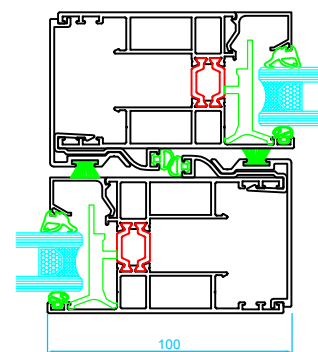
Cruce con refuerzo de inercia estándar
