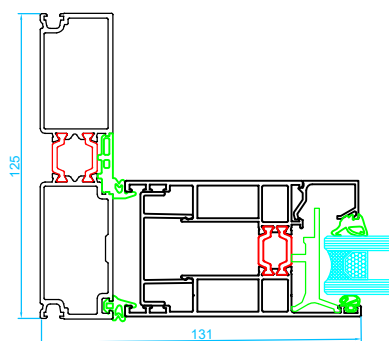
Marco de corredera sección lateral Hoja de corredera
