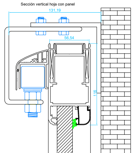
Sección vertical hoja con panel
