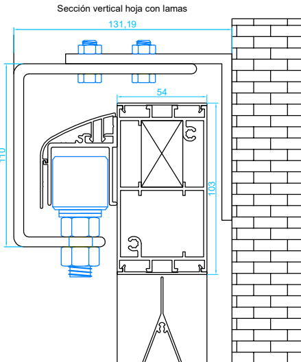
Sección vertical hoja con lamas
