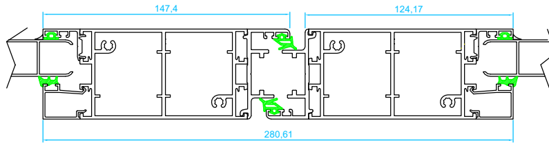
Unión hojas puerta nudo central
